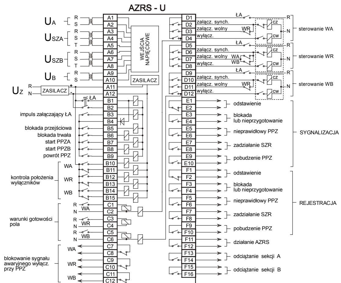
Rys. 7.2.3. Schemat połączeń automatu AZRS-U zasilanego napięciem pomocniczym przemiennym.
