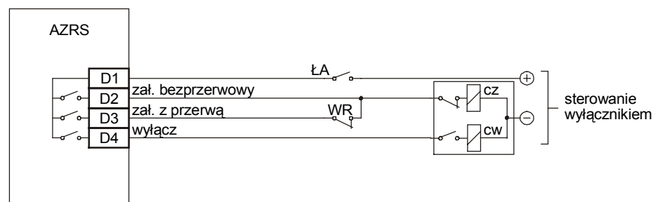
Rys. 7.2.10. Sterowanie wyłącznikiem.
