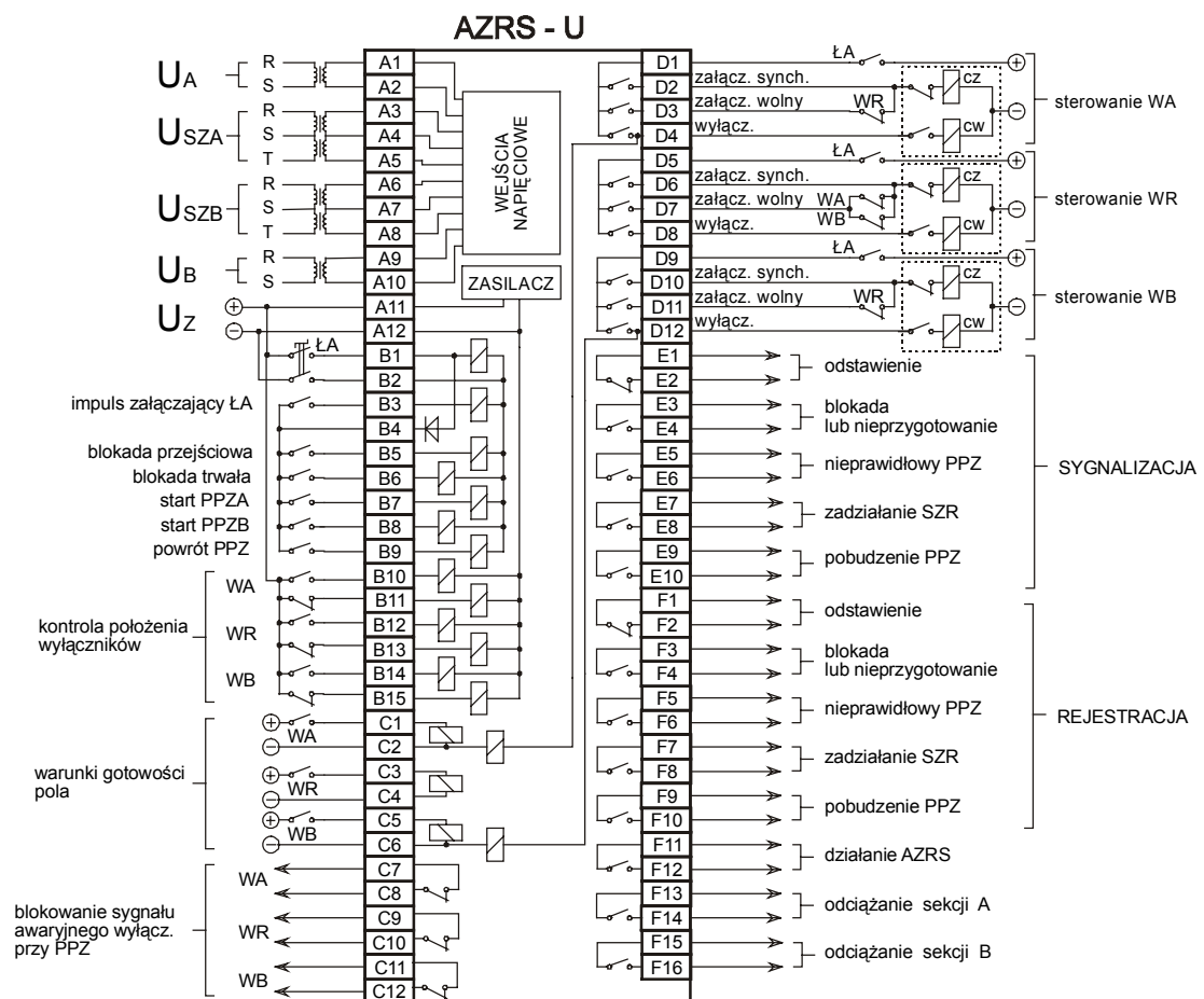
Rys. 7.2. Schemat połączeń automatu AZRS-U w wersji standardowej.
