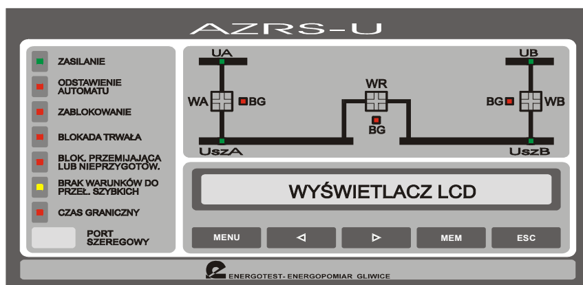
Rys. 3.3. Płyta czołowa automatu.
