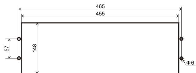
OTWORY W PŁYTCIE MONTAŻOWEJ
