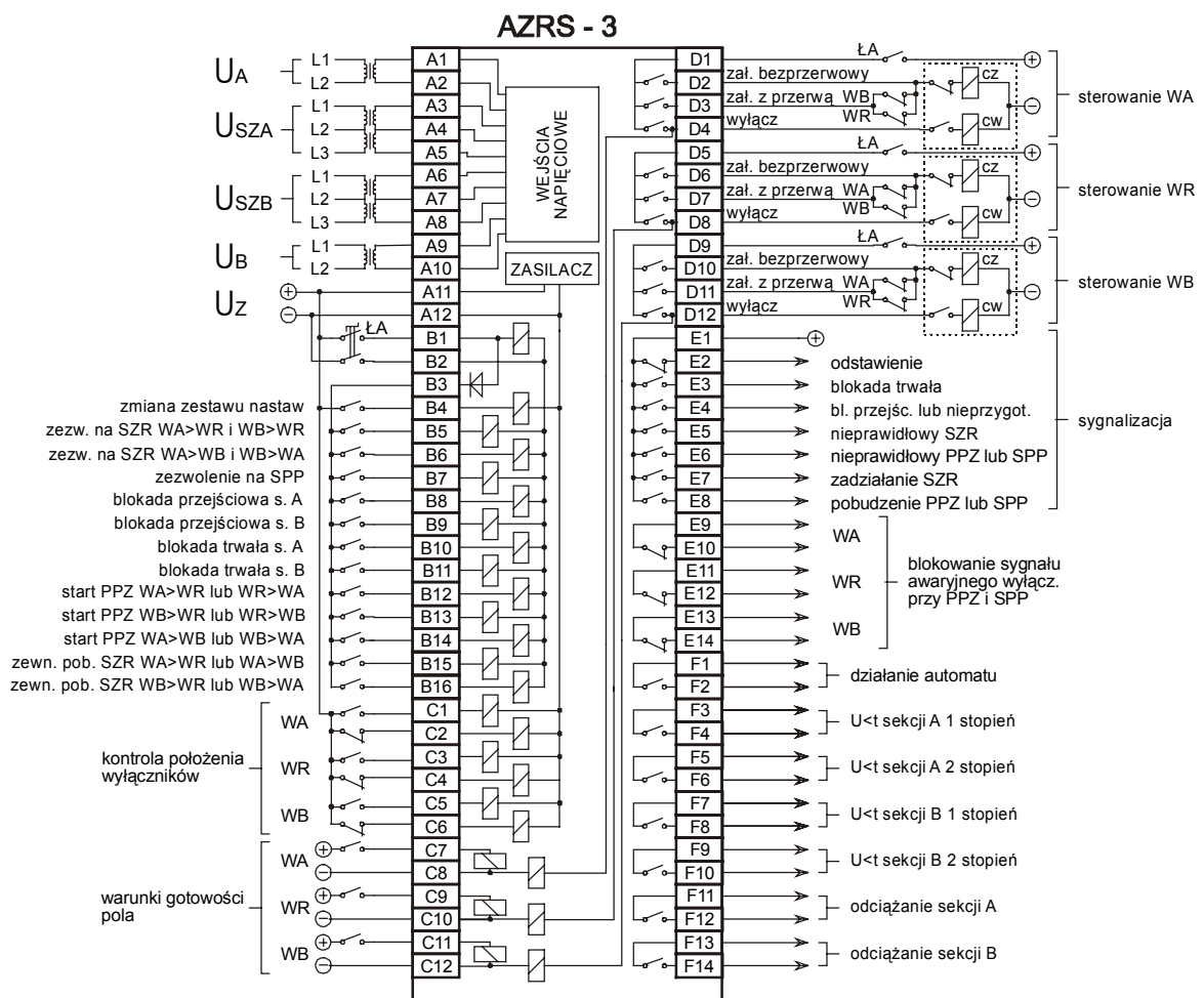
Rys. 7.2. Schemat podłączeń automatu AZRS-3 w wersji standardowej.
