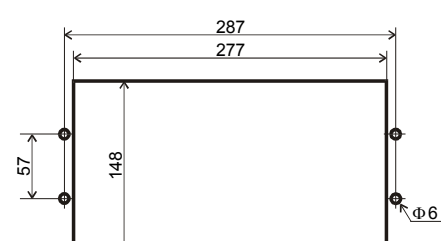
OTWORY W PŁYTCIE MONTAŻOWEJ
