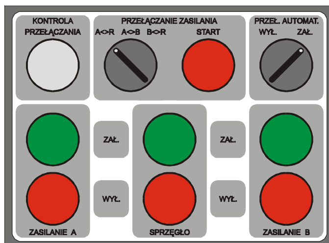
Rys. 7.2.18a. Dodatkowy pulpit.
