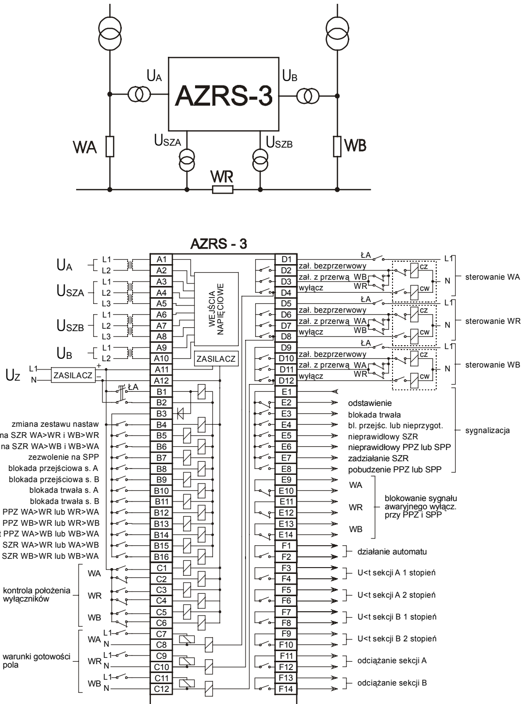
Rys. 7.2.3. Schemat połączeń automatu AZRS-3 zasilanego napięciem pomocniczym przemiennym.
