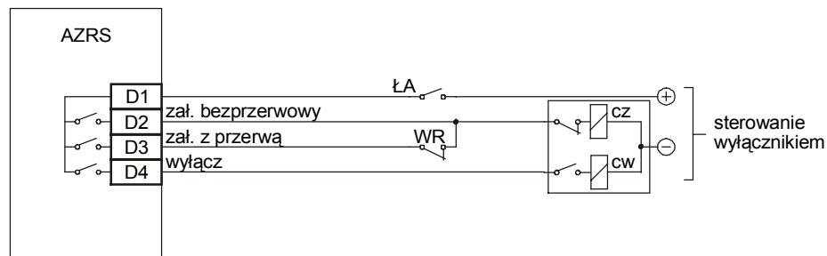
Rys. 7.2.13. Sterowanie wyłącznikiem.
