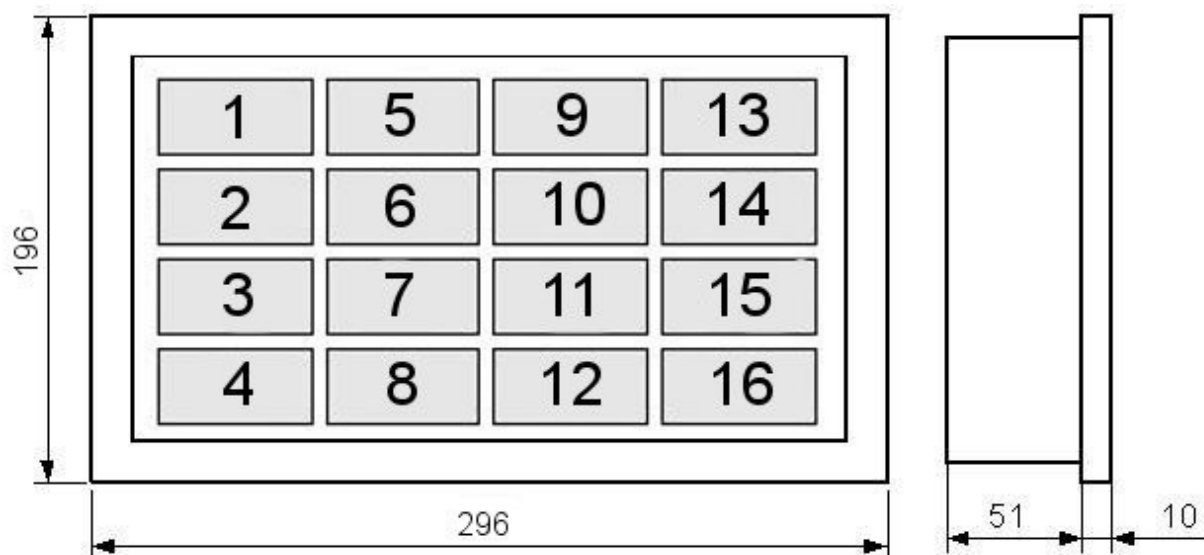
Rys. 1.. Wymiary obudowy i rozmieszczenie pól
