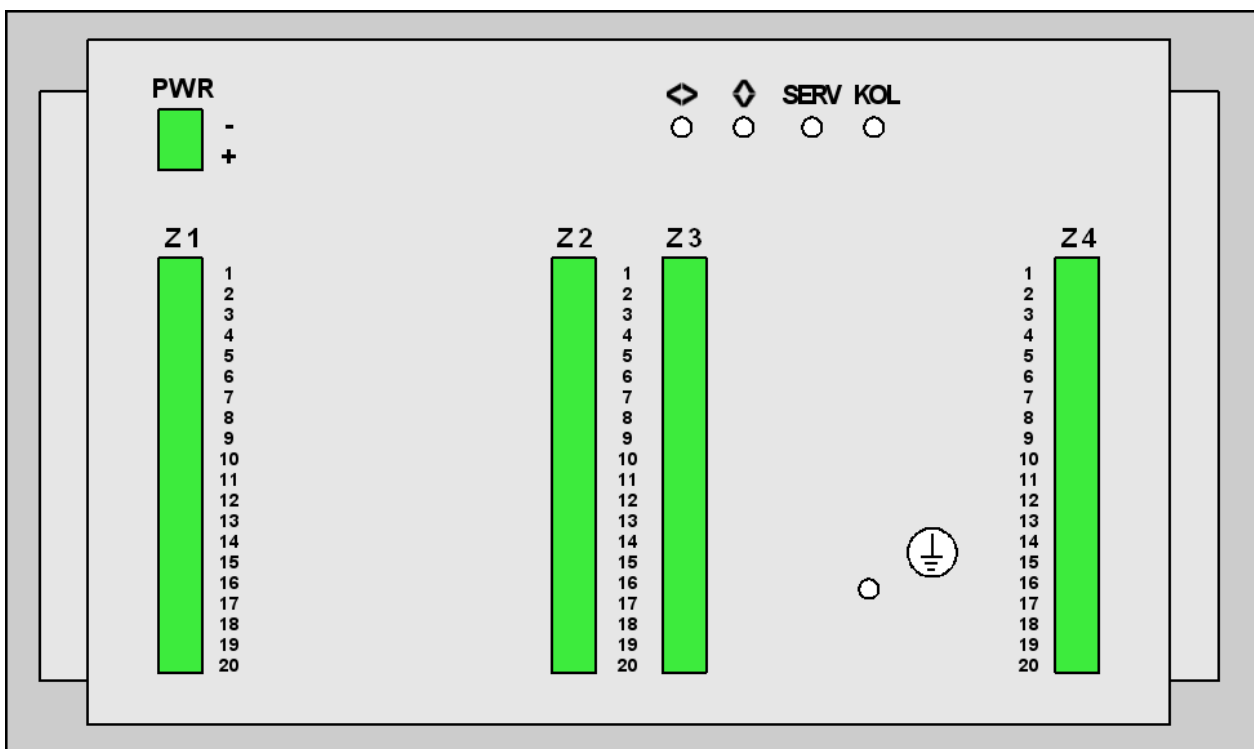
Рис. 3. Вид разъемов
