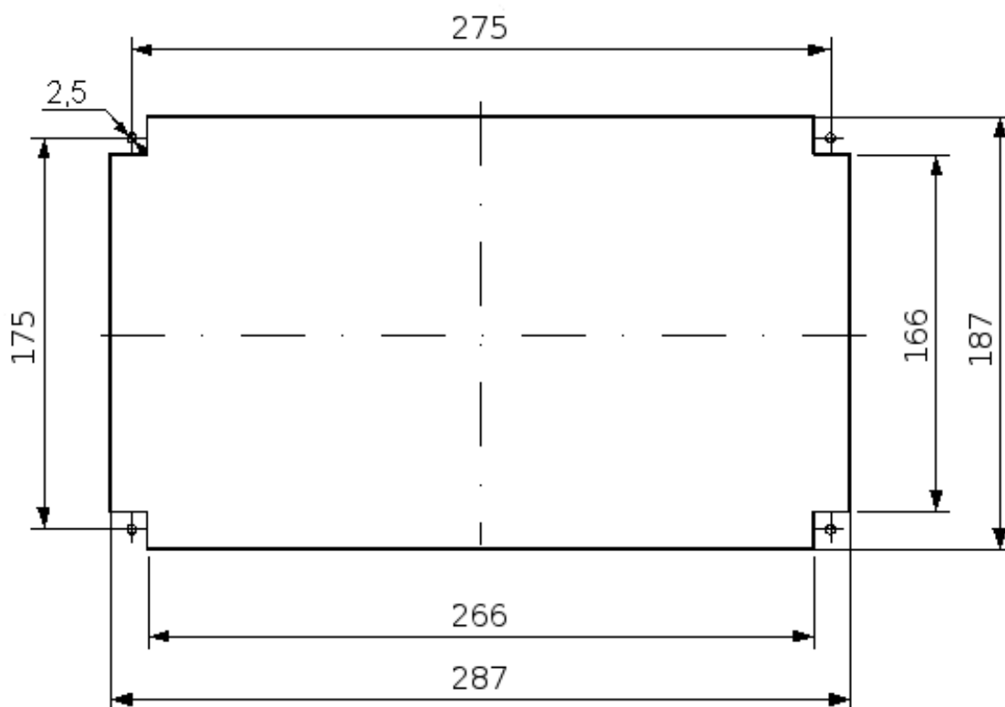
Рис. 2. Монтажное отверстие
