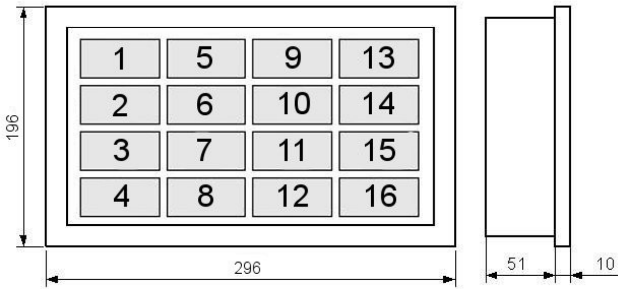
Рис. 1.. Размеры корпуса и размещение полей
