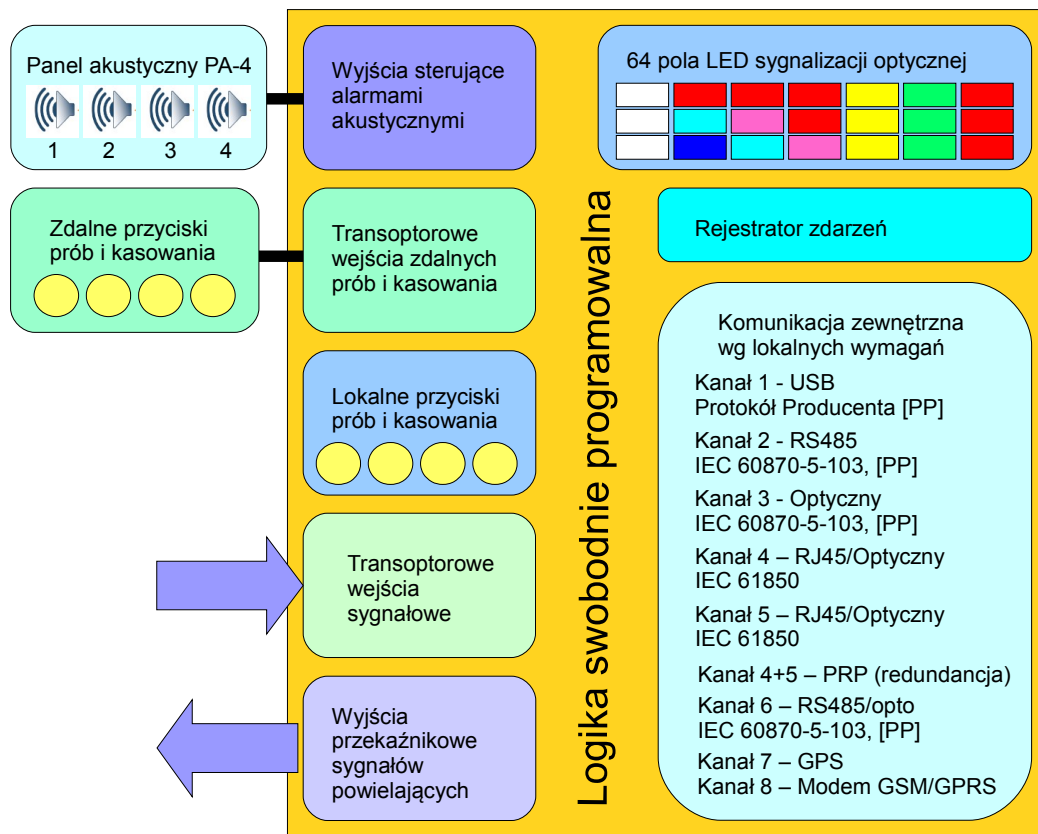
Rys. 4.2: Schemat blokowy.
